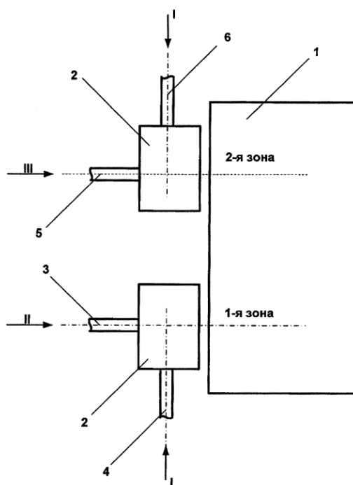
Рисунок 1 – Схема нового двухступенчатого способа сжигания нефтезаводских газов и устройство для его реализации
